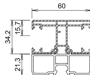
Doppellaufschiene Alu mit Adapter PVC geeignet für Panzer Typ XL 5137 + 5118
