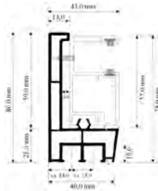
PVC-Führungsschiene 973/933 (bei einteiligen Elementen nur mit versetztem Einlauf der Schienen möglich)
