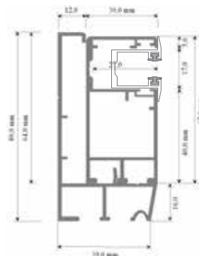
ALU- Führungsschiene
