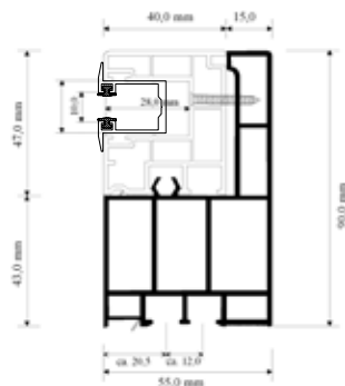
PVC- Führungsschiene 972/930
