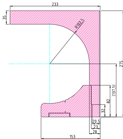
Rolo ISO-TOP RA 26 Variante K
