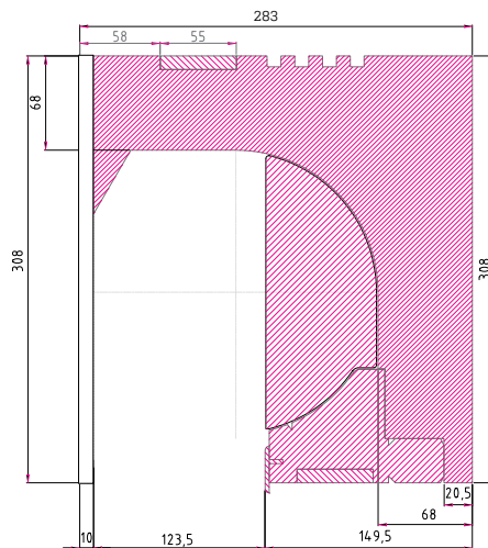
Rolo ISO-TOP Raffstore 30 Variante K-o
