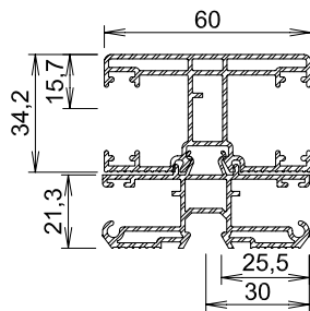
Laufschiene ALU mit Fliegengitterlauf- schiene PVC geeignet für Panzer Typ X PVC 5140 + 5119
