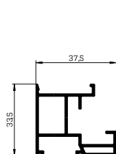
Führungsschiene 2-teilig 3896 (Standard)
