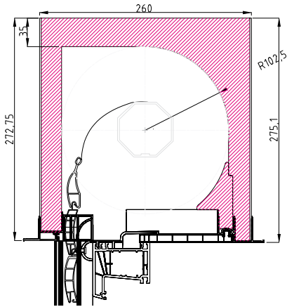
Rolo ISO-TOP RI 26 Variante P
