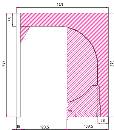
Rolo ISO-TOP Raffstore 26 Variante K-o
