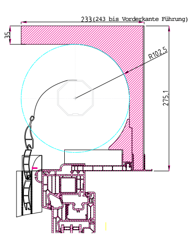
Rolo ISO-TOP RI 26 Variante K
