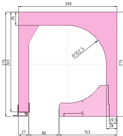
Rolo ISO-TOP RA 26 Variante P
