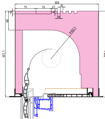
Rolo ISO-TOP RI 30 Variante P
