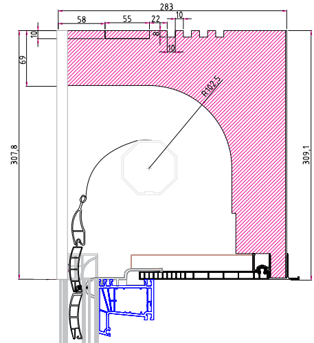
Rolo ISO-TOP RI 30 Variante K-o
