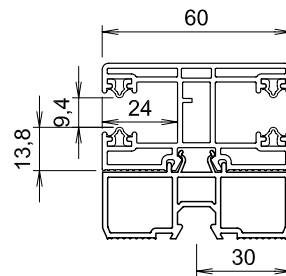
Doppellaufschiene PVC mit Adapter aus PVC geeignet für Panzer Typ X 5117+5118
