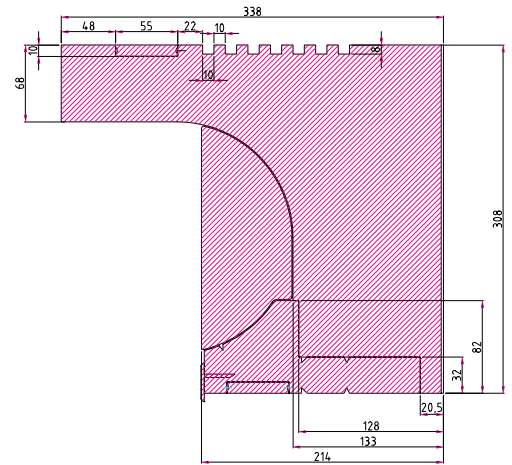
Rolo ISO-TOP Raffstore 36 Variante K
