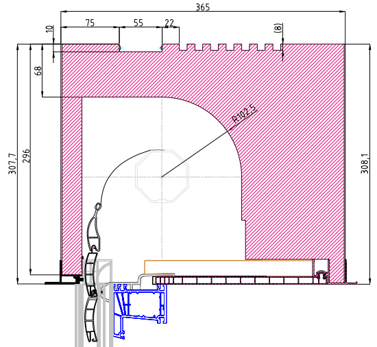
Rolo ISO-TOP RI 36 Variante P
