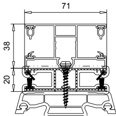
doppelte Insektenschutzfüh- rung (mit doppelter Alu-FS)
