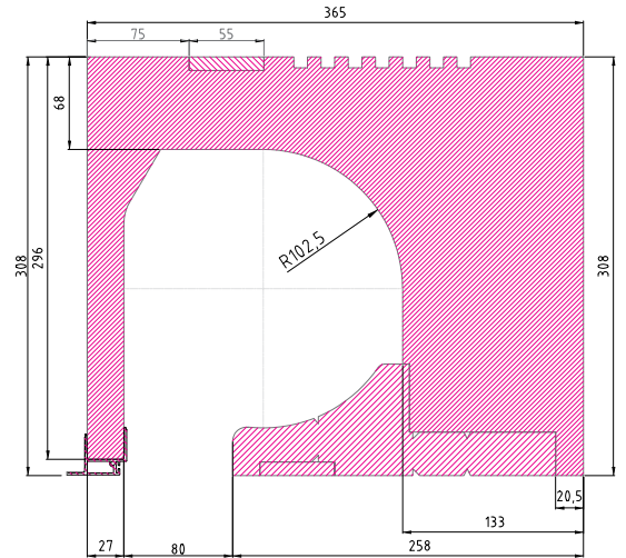
Rolo ISO-TOP RA 36 Variante P
