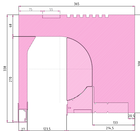
Rolo ISO-TOP Raffstore 36 Variante P
