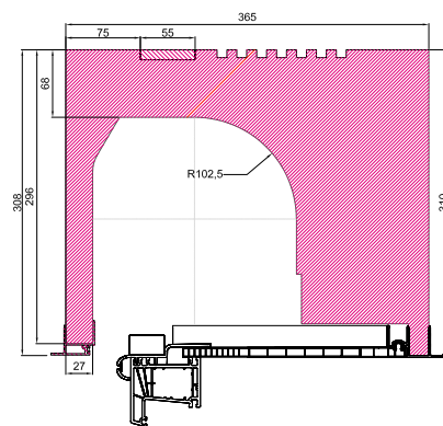
Rolo ISO-BOX 36 Variante P
