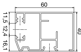
40er ALU-Laufschiene geeignet für TYP X 4142
