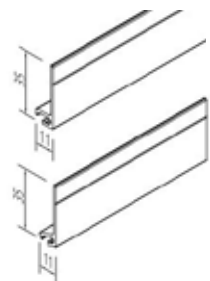
Aufnahmeprofil 90° & 20° – Kombination mit Aluwinkel 20 mm - 80 mm
