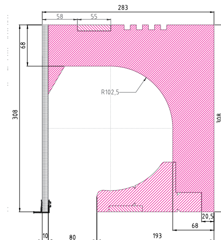
Rolo ISO-TOP RA 30 Variante W
