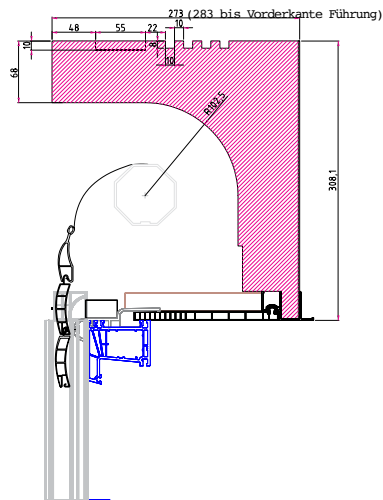
Rolo ISO-BOX 30 Variante K
