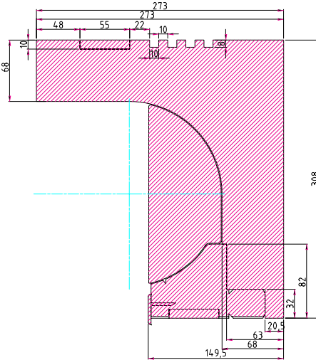
Rolo ISO-TOP Raffstore 30 Variante K
