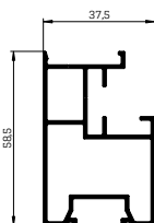
Führungsschienen- aufdopplung 3901
