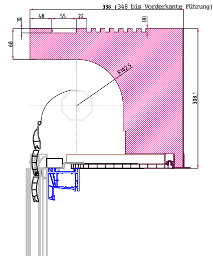
Rolo ISO-BOX 36 Variante K
