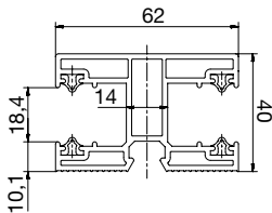
40er PVC-Doppellaufschiene geeignet für TYP XL 4133
