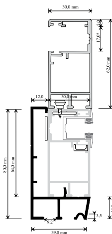
Sonder-Klinker- Führungsschiene PVC
