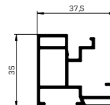
Führungsschiene FMB 3902
