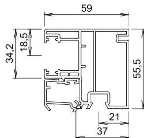
Laufschiene PVC mit Fliegengitterlauf- schiene PVC geeignet für Panzer Typ XL 5116 + 5119
