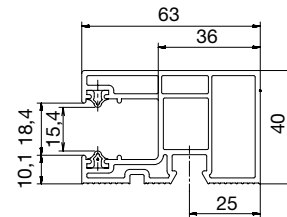
40er PVC-Laufschiene geeignet für TYP XL 4131
