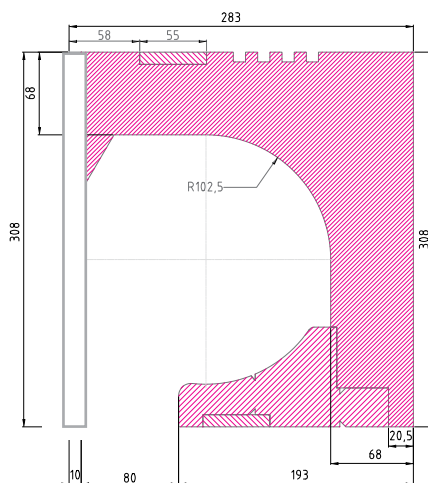
Rolo ISO-TOP RA 30 Variante K-o
