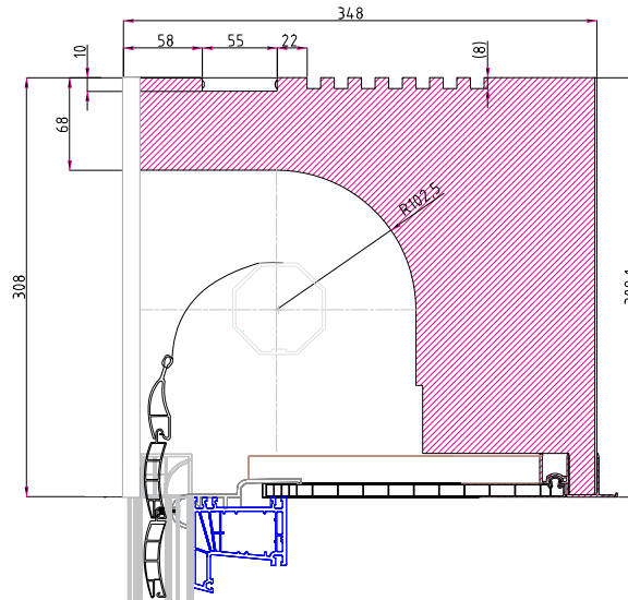
Rolo ISO-TOP RI 36 Variante K-o
