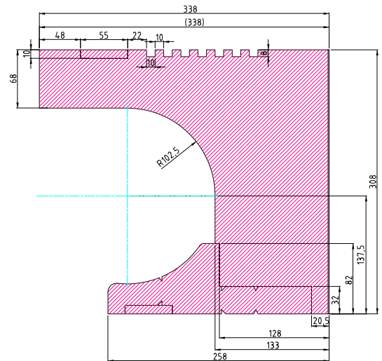
Rolo ISO-TOP RA 36 Variante K
