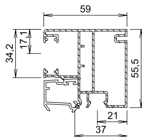
Laufschiene Alu mit Fliegengitterlauf- schiene PVC geeignet für Panzer Typ XL 5141 + 5119
