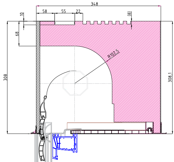
Rolo ISO-TOP RI 36 Variante W
