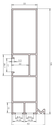
Sonder-Klinker- Führungsschiene ALU
