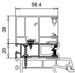
Insektenschutzführung (mit Alu-FS)
