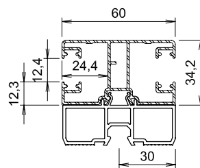
Doppellaufschiene Alu mit Adapter PVC geeignet für Panzer Typ X 5197 + 5118
