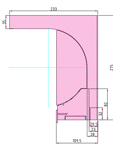
Rolo ISO-TOP Raffstore 26 Variante K
