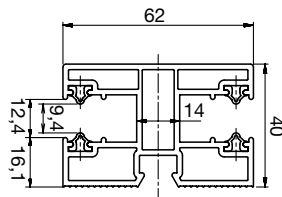
40er PVC-Doppellaufschiene geeignet für TYP X 4132
