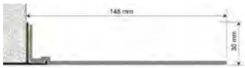
10025 – Putzwinkelverlängerung, zuschneidbar in 5 mm Schritten Preis 6,95 €/m
