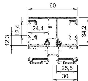
Doppellaufschiene Alu mit Insektenschutz Adapter Alu geeignet für Panzer Typ X 5197 + 5138
