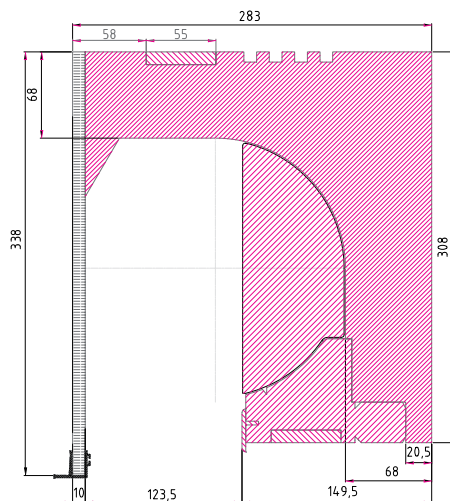
Rolo ISO-TOP Raffstore 30 Variante W
