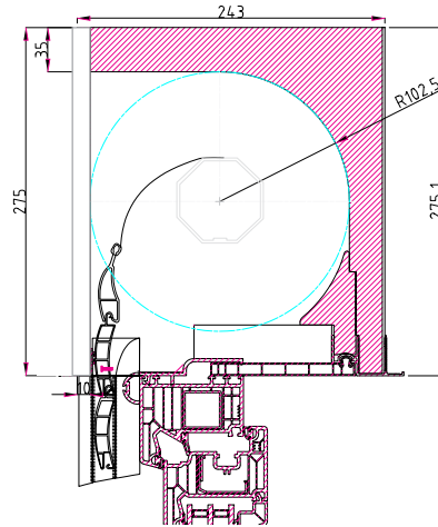
Rolo ISO-TOP RI 26 Variante K-o
