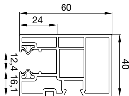
40er PVC-Laufschiene geeignet für TYP X 4130
