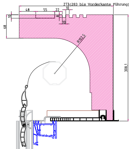
Rolo ISO-TOP RI 30
