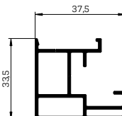
Führungsschiene VS Z contra 3899
