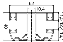
40er ALU-Doppellaufschiene geeignet für TYP X 4143
