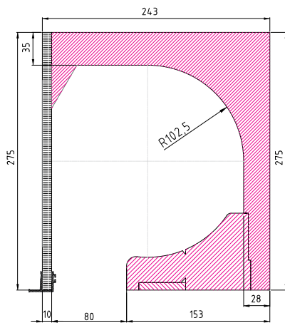
Rolo ISO-TOP RA 26 Variante W
