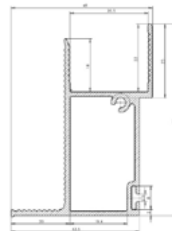
Putzwinkel ALU Außen - 26er Schachthöhe
