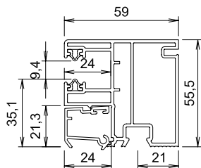
Laufschiene PVC mit Fliegengitterlauf- schiene PVC geeignet für Panzer Typ X 5115 + 5119
