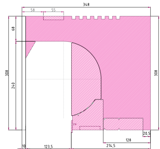
Rolo ISO-TOP Raffstore 36 Variante K-o
