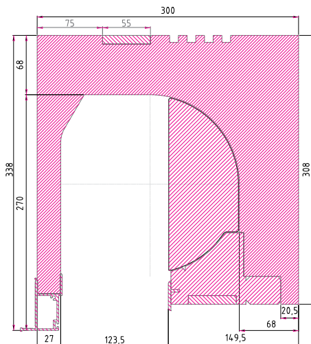
Rolo ISO-TOP Raffstore 30 Variante P
