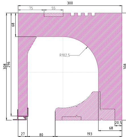
Rolo ISO-TOP RA 30 Variante P
