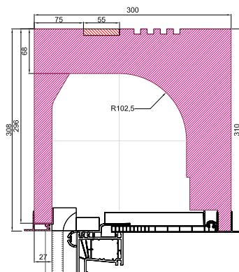
Rolo ISO-BOX 30 Variante P
