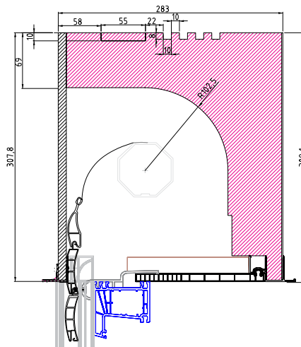
Rolo ISO-TOP RI 30 Variante W
