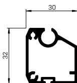
Endleiste Typ 1 3907 (Standard bis 350 cm Elementbreite)
