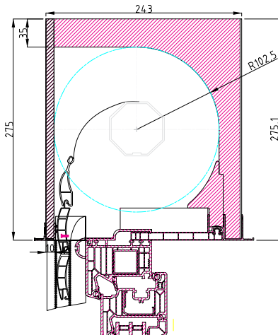
Rolo ISO-TOP RI 26 Variante W
