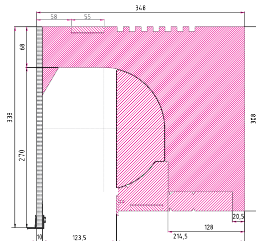
Rolo ISO-TOP Raffstore 36 Variante W
