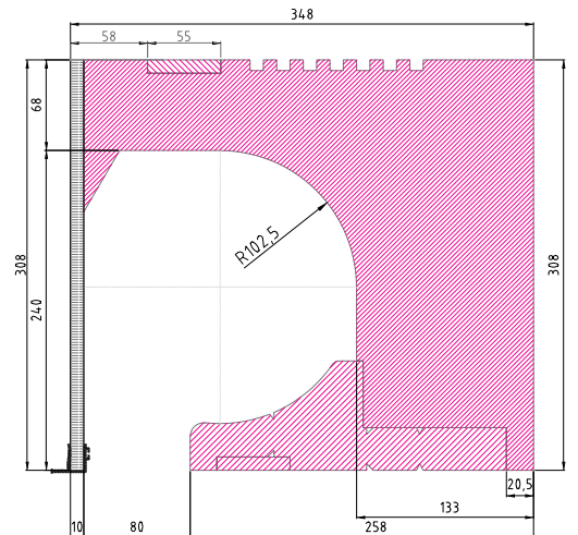
Rolo ISO-TOP RA 36 Variante W
