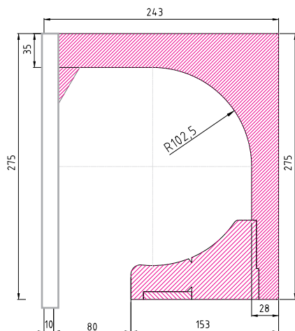
Rolo ISO-TOP RA 26 Variante K-o
