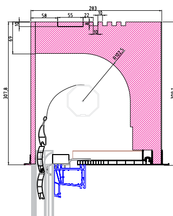
Rolo ISO-BOX 30 Variante W
