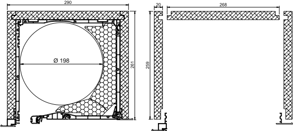
5047 Alu-Putz-schiene außen
