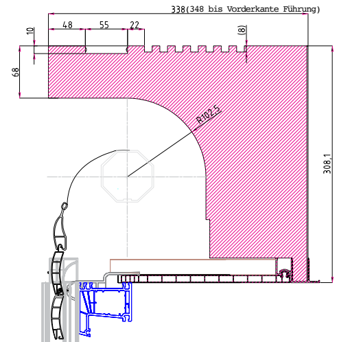
Rolo ISO-TOP RI 36 Variante K
