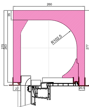
Rolo ISO-BOX 26 Variante P
