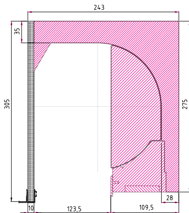
Rolo ISO-TOP Raffstore 26 Variante W
