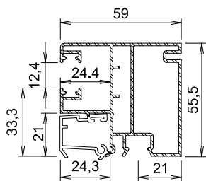
Laufschiene PVC mit Fliegengitterlauf- schiene PVC geeignet für Panzer Typ X 5115 + 5119
